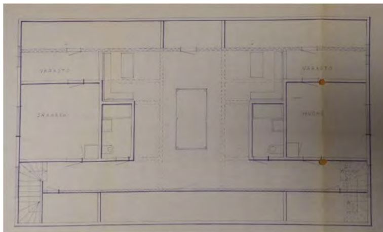
Tallihovin toisen kerroksen muutospirustus vuodelta 1973. (Lappeenrannan rakennusvalvonta)
