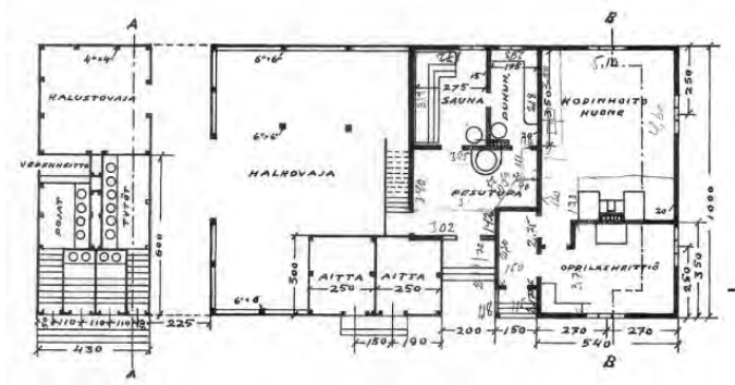
Vuonna 1937 valmistuneen talousrakennuksen pohjapiirros. (Lappeenrannan tilakeskus)
