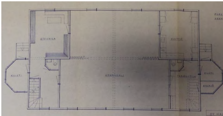
Tallihovin muutospiirustus vuodelta 1973, joka vastaa Mälkniemen pohjakaavaa. (Lappeenrannan rakennusvalvonta)
