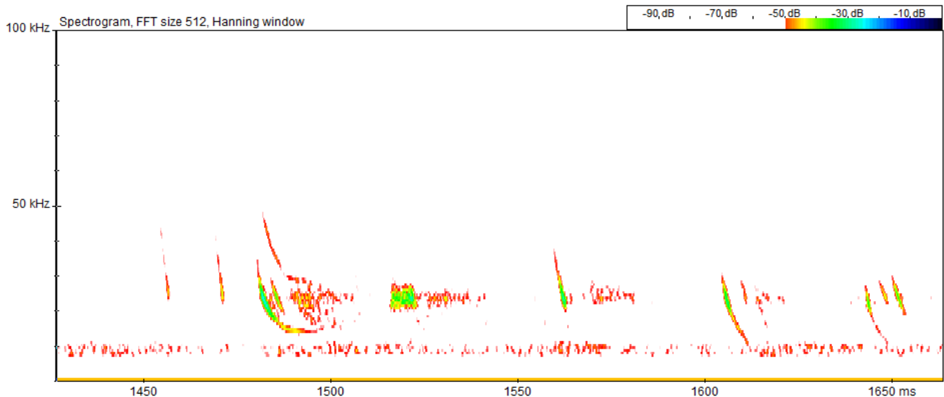
Kuva 3. Esimerkki pohjanlepakon sosiaalisista äänistä Lappeenrannan Honkalahden selvitys-alueella 30.8.2017 BatSound 4.1 -ohjelmalla esitettyinä. Pystyakseli kuvaa taajuutta kilohertseinä (kHz) ja vaaka-akseli aikaa (mittaväli 50 ms).
