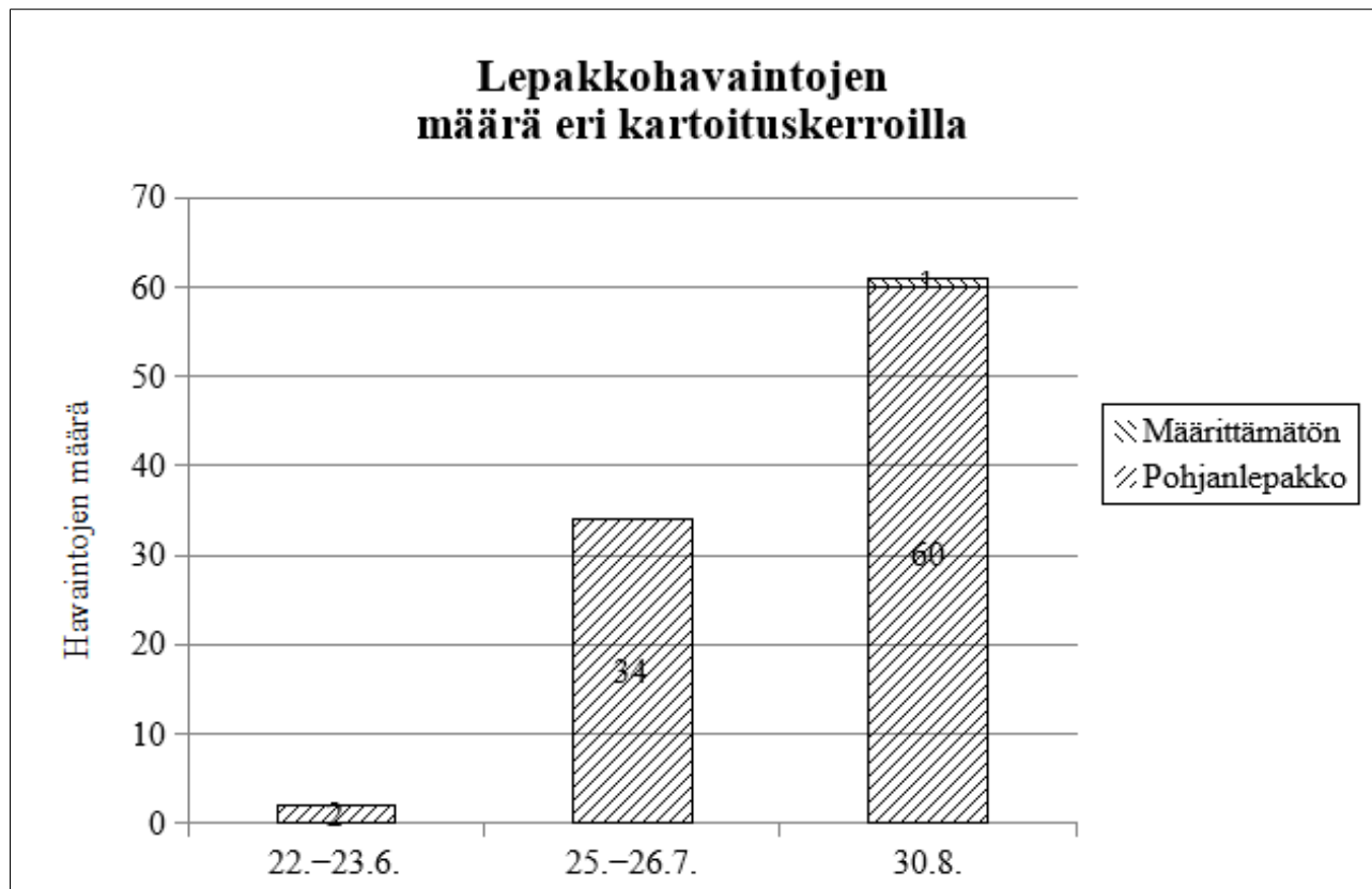
Kuva 4. Lepakkohavaintojen määrä kolmella eri kartoituskerralla Lappeenrannan Honkalahden lepakkoselvityksessä 22.6.–30.8.2017.
