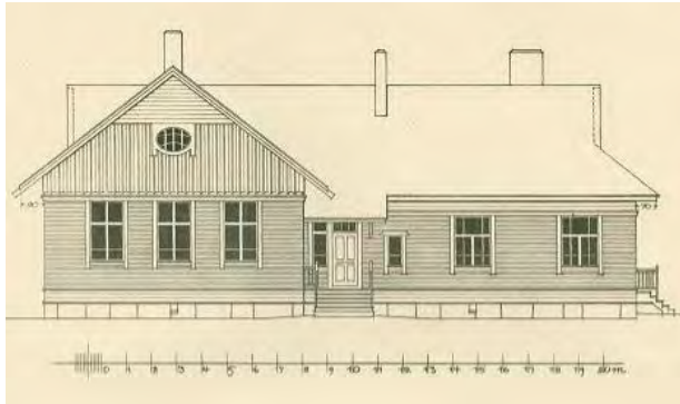
Tyyppipiirustus no 9. (ELKA)
