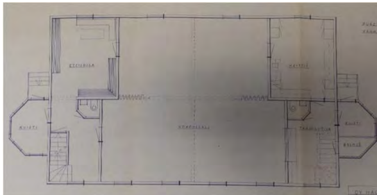
Tallihovin ensimmäisen kerroksen muutospirustus vuodelta 1973. (Lappeenrannan rakennusvalvonta)
