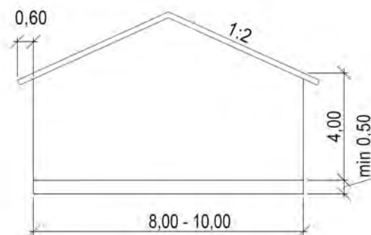
Kuva 1. Rakennuksen suositeltavat mitasuhteet.
