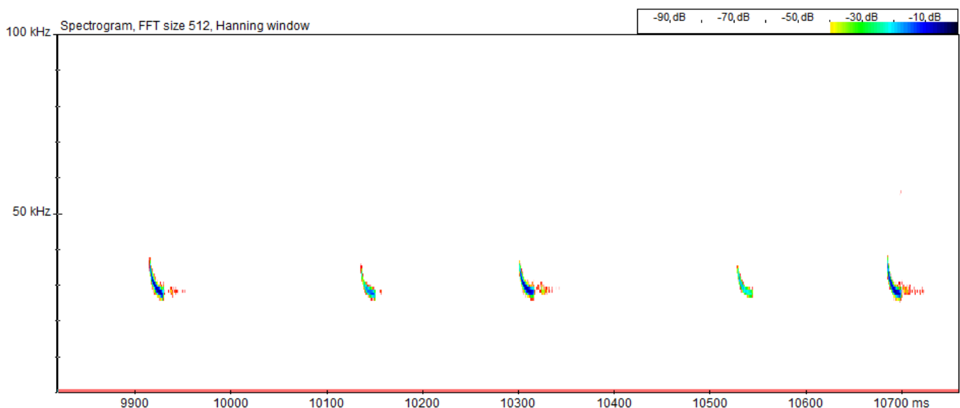
Kuva 2. Esimerkki aukealla saalistavan pohjanlepakon ( Eptesicus nilssoni ) kaikuluotausäänistä Lappeenrannan Honkalahden selvitysalueella 30.8.2017 BatSound 4.1 -ohjelmalla esitettynä. Pystyakseli kuvaa taajuutta kilohertseinä (kHz) ja vaaka-akseli aikaa (mittaväli 100 ms).
