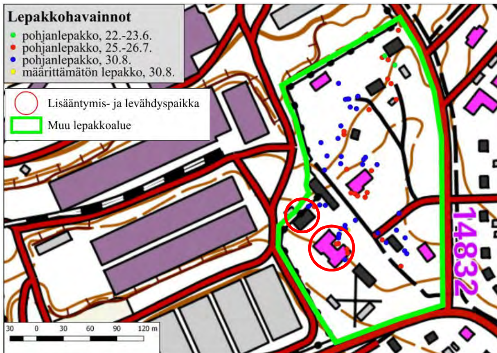
Kuva 18. Lepakko havainnot, lepakoiden lisääntymis- ja levähdyspaikkoina käyttämät rakennukset ja muun huomionarvoisen lepakkoalueen raja. Kuva: Kuitunen 2018, muokattu.
